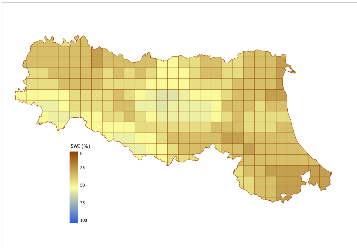
Figura 7 - Soil Water Index sul territorio regionale, risoluzione 12 km. La mappa rappresenta i valori medi di SWI sul periodo di riferimento.
