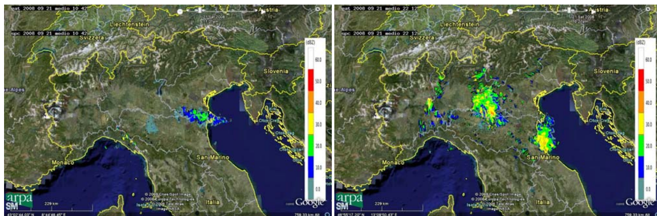
Mappa di riflettività del 21/09/2008 alle 10:42 e alle 22:12 UTC
