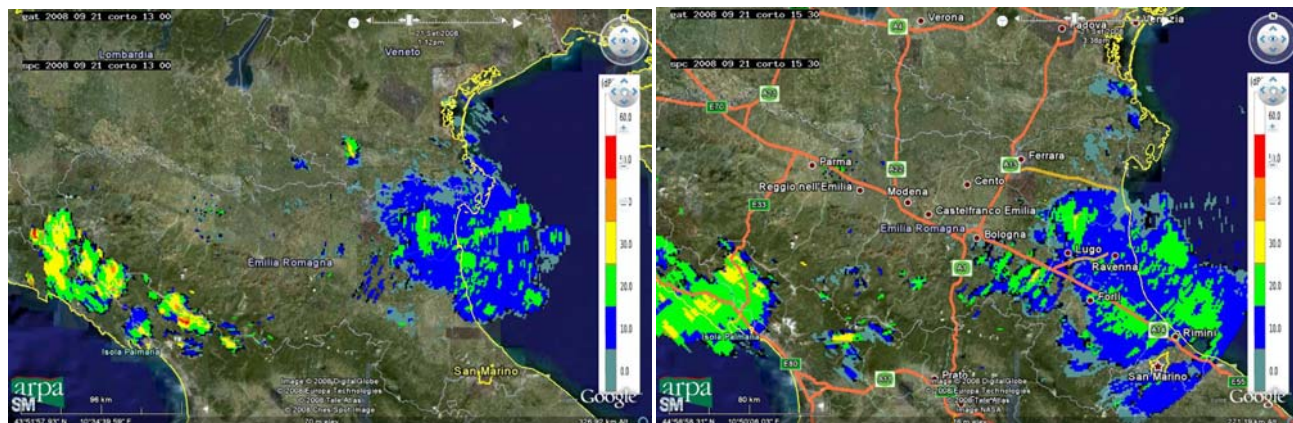
Mappa di riflettività del 21/09/2008 alle 13:00 e alle 15:30 UTC
