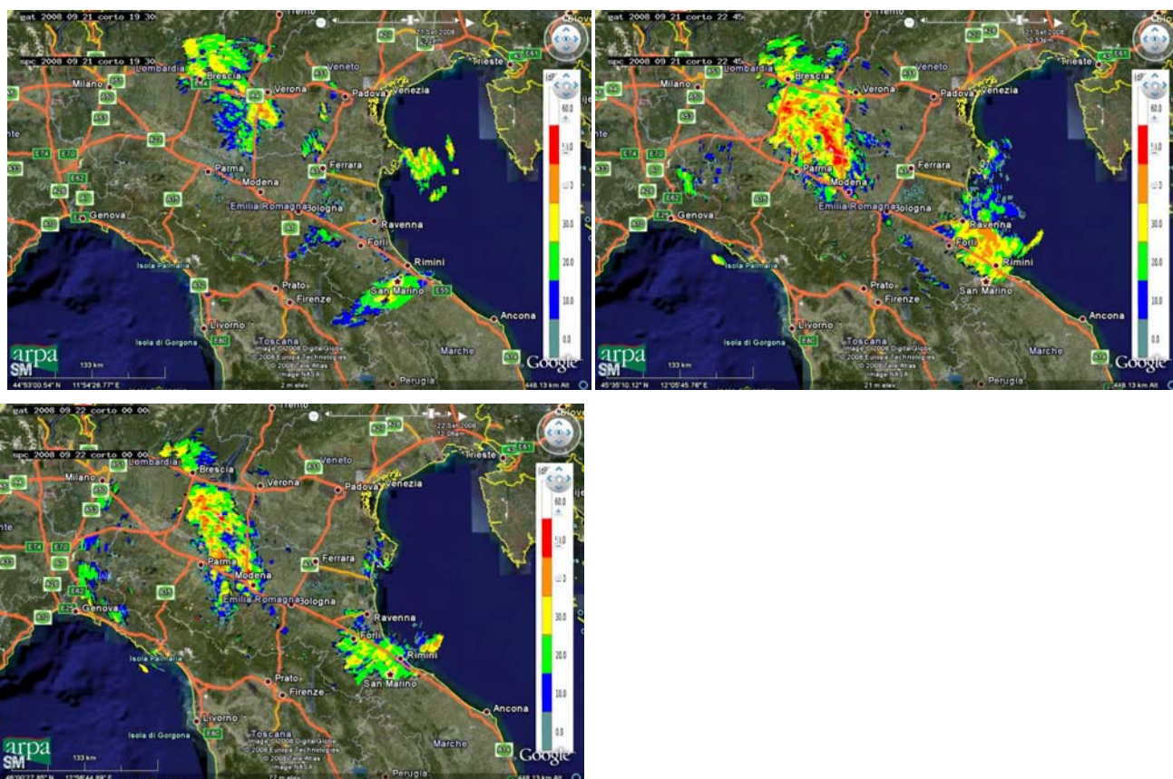
Mappa di riflettività del 21/09/2008 alle 19:30 (alto a sinistra), 22:45 (alto a destra) UTC e del 22/09/2008 alle 00:00 UTC (basso a sinistra)
