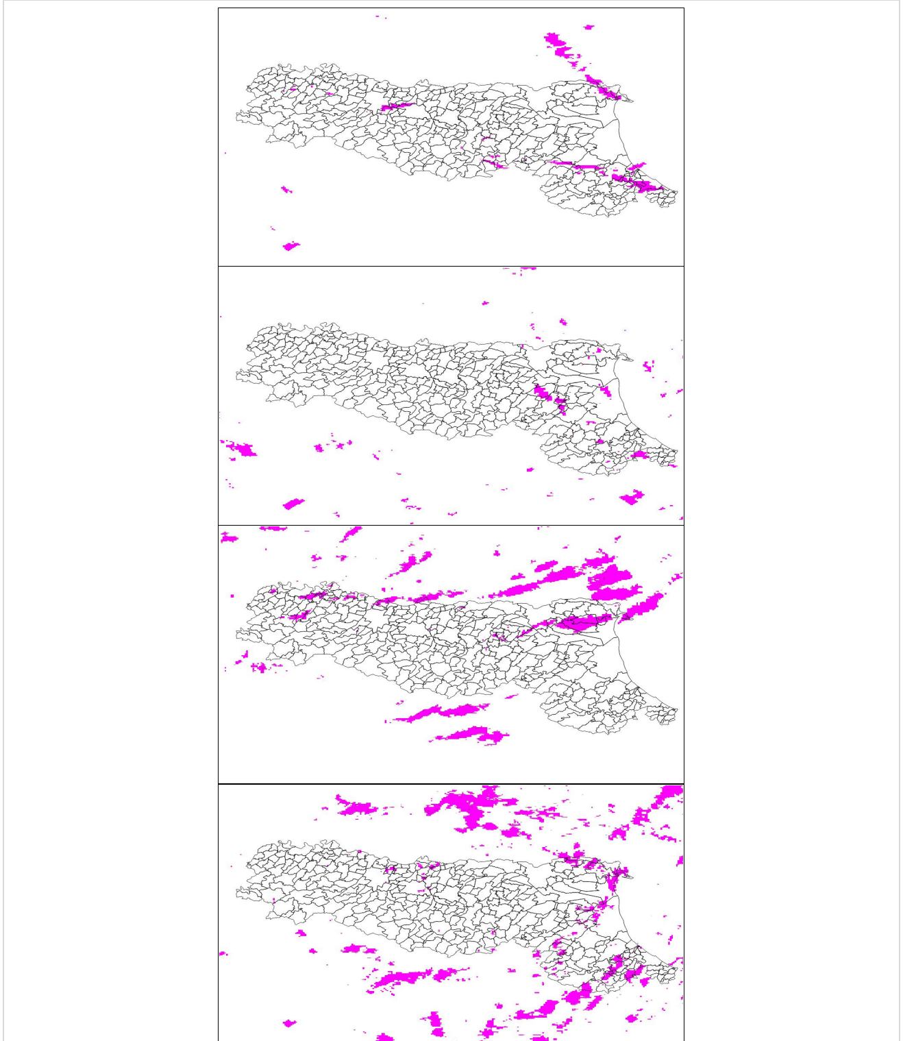
Figura 16. Mappe giornaliere di probabilità di grandine > 99% del 31/8/2018 (in alto), del 1/9 (al centro, sopra), del 2/9/2018 (al centro,sotto) e del 3/9 (in basso) .
