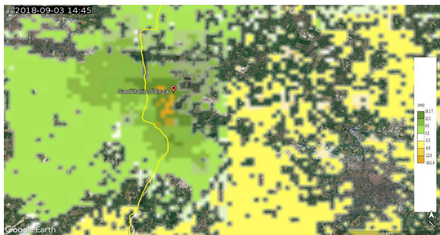
Figura 27. Mappa di vento radiale dal radar di Gattatico del 03/09/2018 alle 14:45 UTC, zoom sull'area di Sant'Ilario d'Enza.
