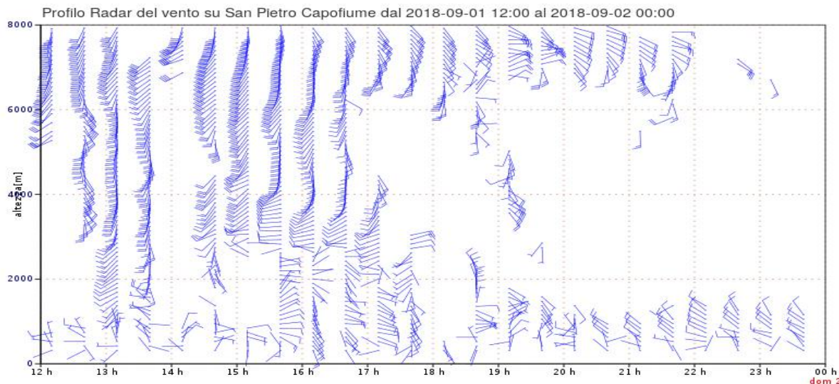
Figura 22. Profilo verticale del vento ottenuto tramite tecnica VAD sui dati del radar di San Pietro Capofiume dalle 12 UTC del 01/09/2018 alle 00 UTC del 02/09/2018
