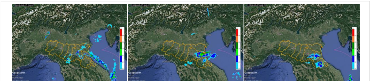
Figura 5. Cumulate orarie stimate dal composito radar del Dipartimento di Protezione civile Nazionale sul Nord Italia del 14/08/2018 alle 11 UTC (a sinistra), alle 15 UTC (al centro) ed alle 19 UTC (a destra).
