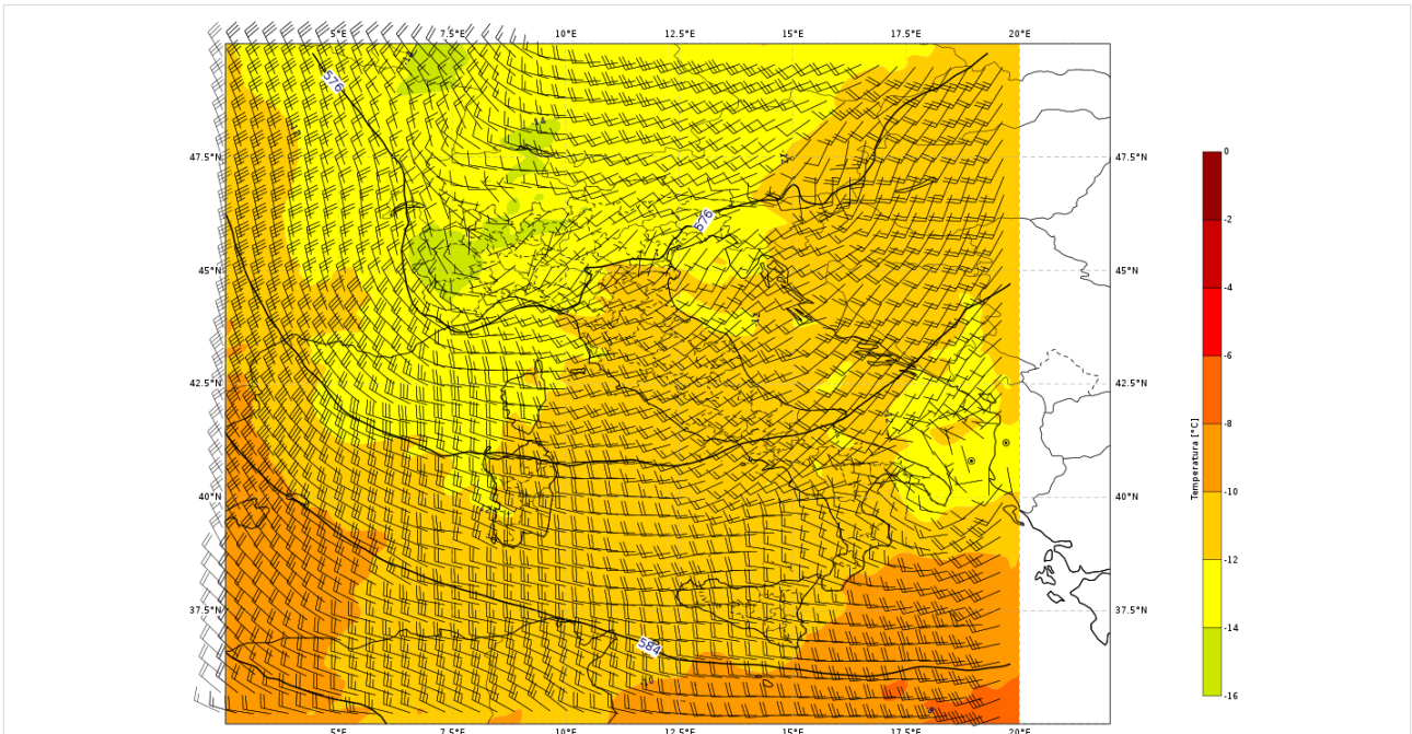
Figura 3. Mappa di analisi (da modello IFS-ECMWF) di geopotenziale, temperatura e vento a 500 hPa del 14/08/2018 alle 12 UTC, centrata sull'Italia.
