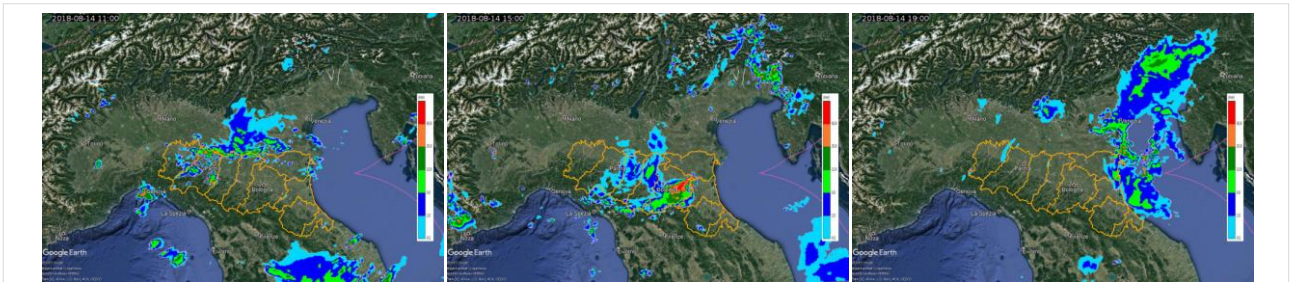
Figura 4. Cumulate orarie stimate dal composito radar del Dipartimento di Protezione civile Nazionale sul Nord Italia del 14/08/2018 alle 11 UTC (a sinistra), alle 15 UTC (al centro) ed alle 19 UTC (a destra).
