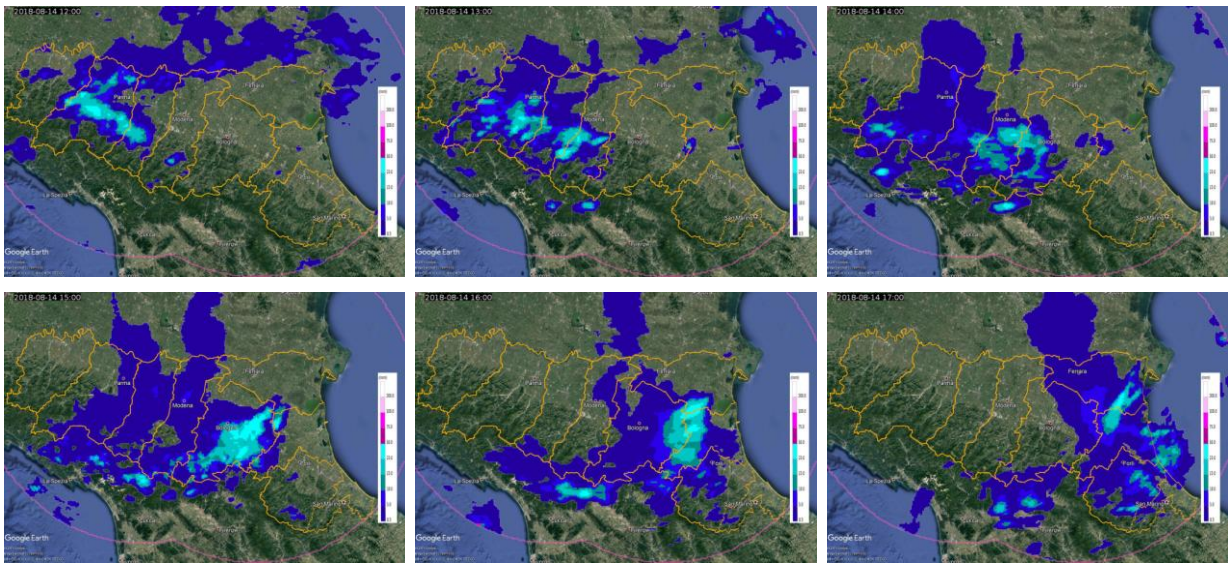
Figura 36. Sequenza di cumulate orarie stimate dal composito radar del 14/08/2018 dalle 12 UTC (in alto a sinistra) alle 17 UTC (in basso a destra).
