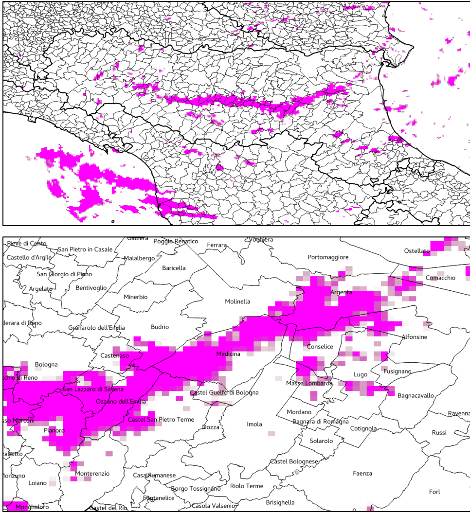
Figura 50. Probabilità di grandine superiore al 99%, stimata da radar, per la giornata del 14/08/2018 (in alto) e zoom sulle aree che hanno registrato i maggiori disagi a seguito del passaggio dei fenomeni precipitanti (in basso).
