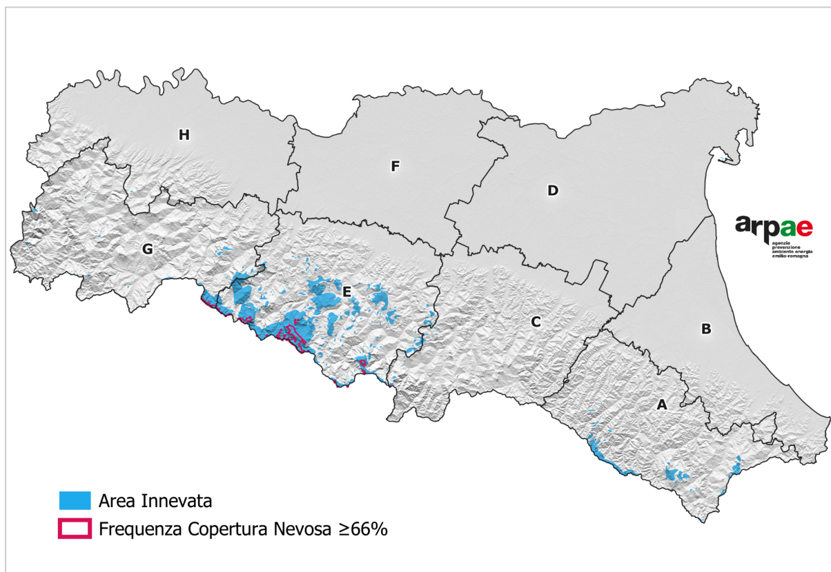
Figura 5 - Mappa dell'innervamento da dati satellitari e modellistici sulle macroaree omogenee dal punto di vista climatologico e idrologico della Regione Emilia-Romagna. La presenza di copertura nevosa viene mostrata in azzurro, mentre i contorni di colore rosso rappresentano le zone in cui, nell'intervallo di riferimento 2000 - 2023, è stata rilevata la presenza di neve con frequenza maggiore o uguale al 66% nella metà del mese in cui ricade l'immagine satellitare del presente bollettino.
