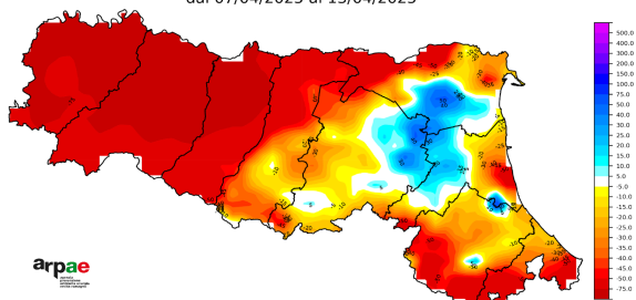
Anomalia percentuale delle precipitazioni settimanali dal 07/04/2025 al 13/04/2025
