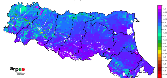
Frazione di acqua disponibile nel suolo 13/04/2025
