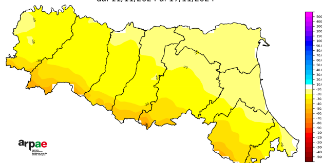
Anomalia delle precipitazioni settimanali dal 11/11/2024 al 17/11/2024
