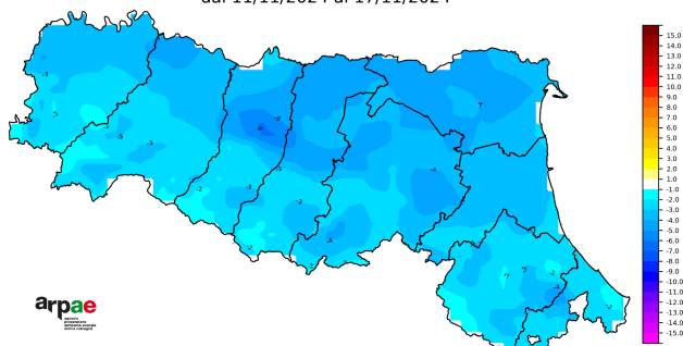
Anomalia delle temperature minime dal 11/11/2024 al 17/11/2024
