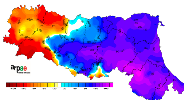
Anomalia del Bilancio Idroclimatico (mm) dal 01/01/2023 al 28/05/2023
