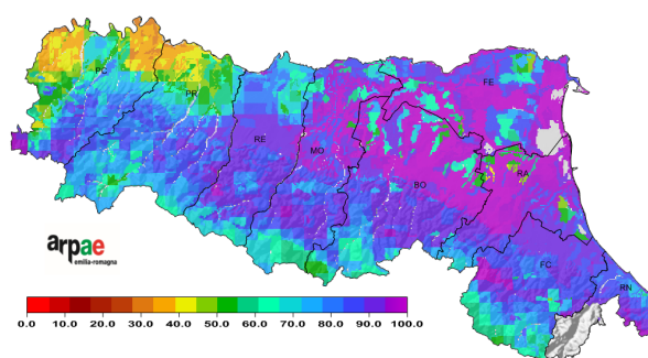
Percentile di Acqua disponibile (U-PA) (-) al 28/05/2023 Condizione Culturale: Prato di graminacee
