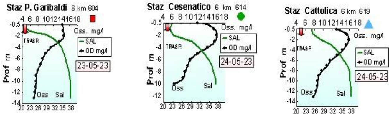
Figura 14 – Profili di salinità (psu) e ossigeno disciolto (mg/l) eseguiti con sonda multiparametrica durante i controlli del 22-23-24 Maggio nelle stazioni a 6 km prospicienti Porto Garibaldi, Cesenatico e Cattolica
