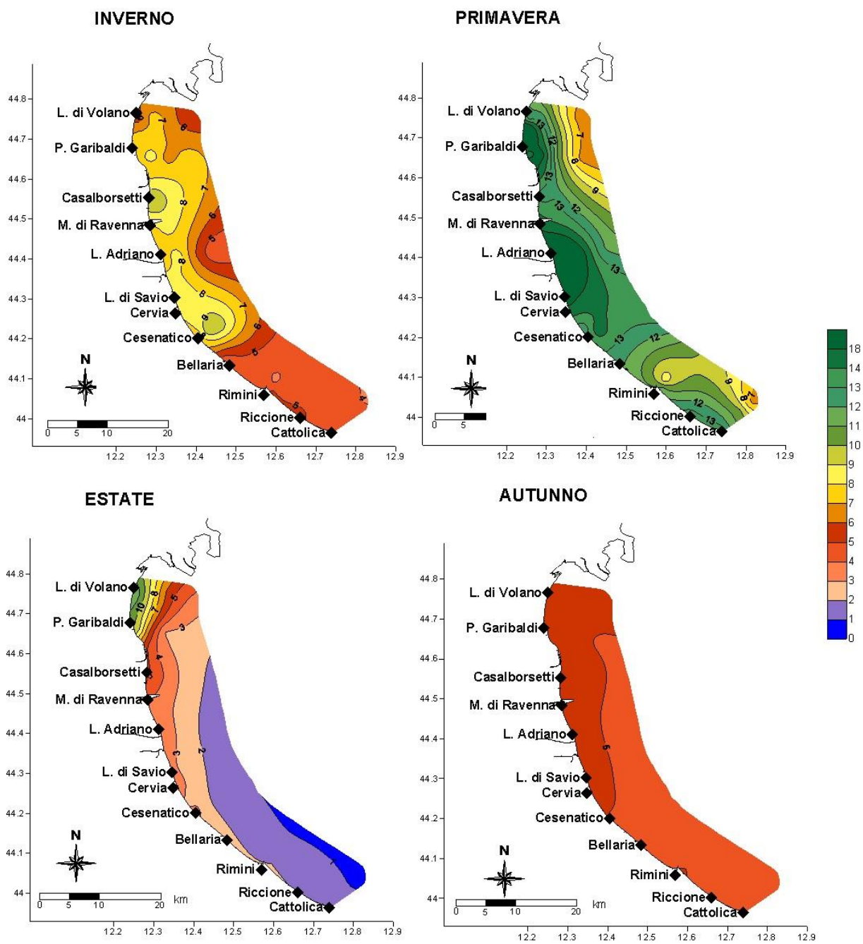
Figura 56 – Mappe di distribuzione della clorofilla “a” ( \mu\text{g/l} ) da costa a 10 km al largo in superficie (medie stagionali 2023)
