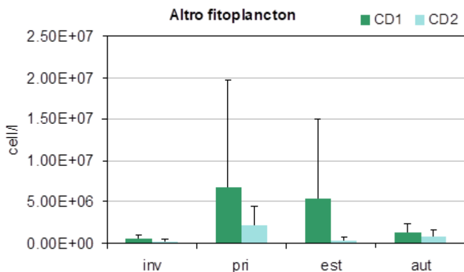
Figura 119 - Andamento delle medie stagionali e deviazioni standard dell'Altro fitoplancton nei corpi idrici CD1 e CD2
