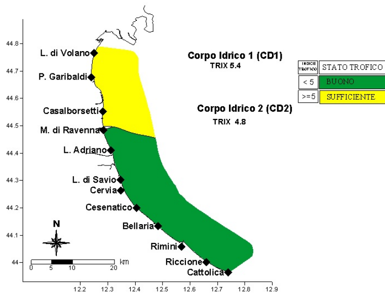
Figura 102 – Valori medi annuali 2023 di TRIX nei due corpi idrici
