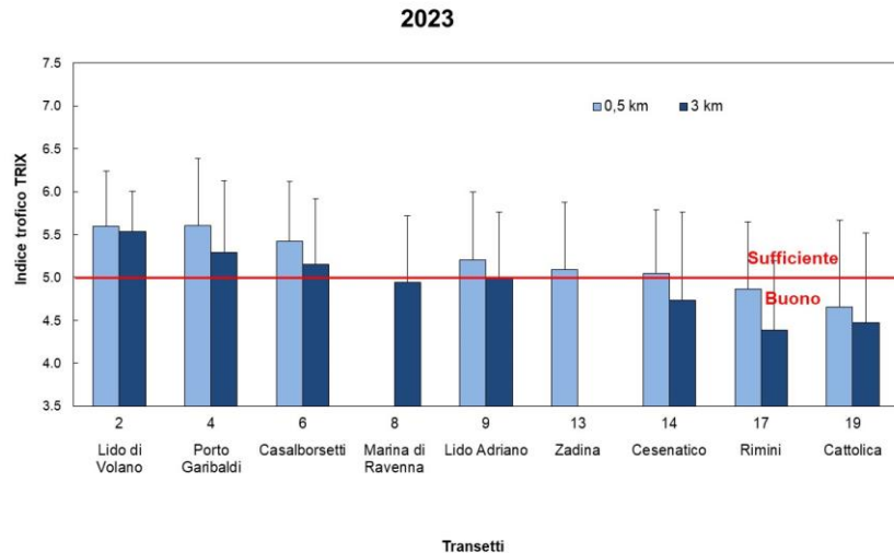
Figura 101 – Medie annuali del TRIX nel 2023 nelle stazioni a 0.5 e 3 km dalla costa
