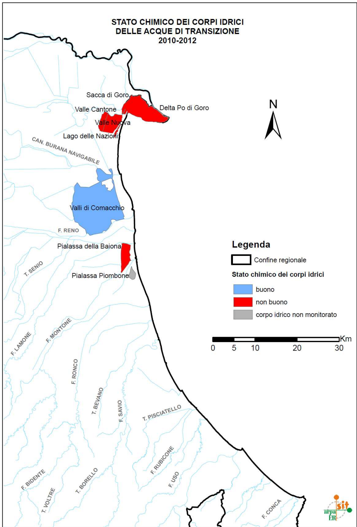
Figura 59 - Stato chimico delle acque di transizione: triennio 2010-2012
