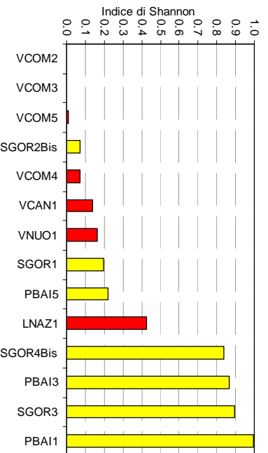
Figura 11 - Indice di Shannon per campagna di monitoraggio (lagune aperte ■ , lagune chiuse ■ ): 2011
