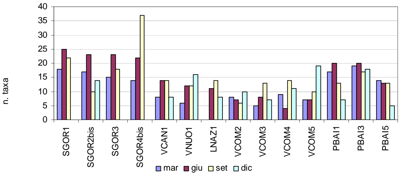
Figura 5 - Numero di taxa per campagna di monitoraggio: 2011
