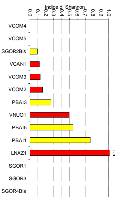
Figura 11 - Indice di Shannon per campagna di monitoraggio (lagune aperte ■ , lagune chiuse ■ ): 2011
