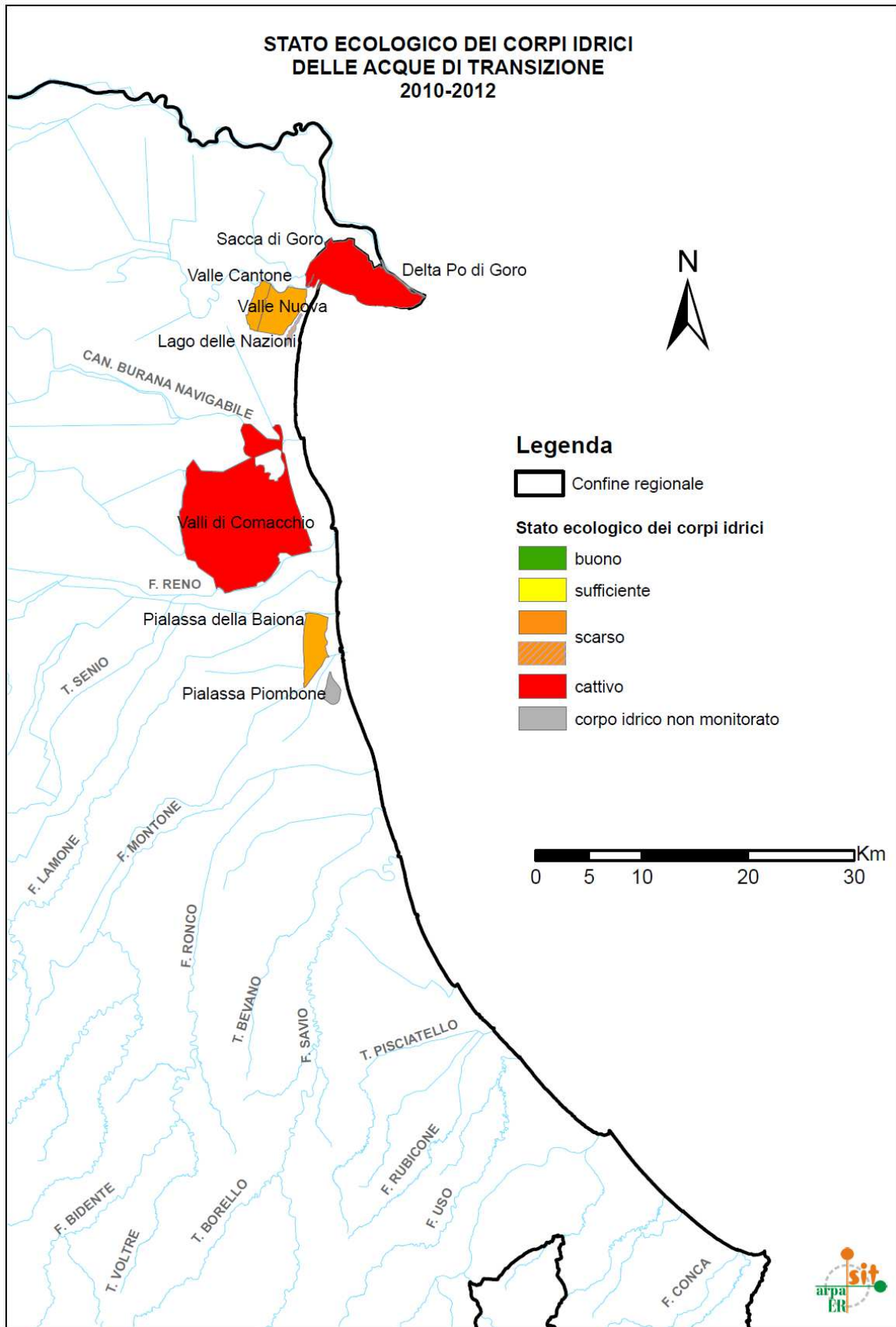
Figura 58 - Stato ecologico delle acque di transizione: triennio 2010-2012
