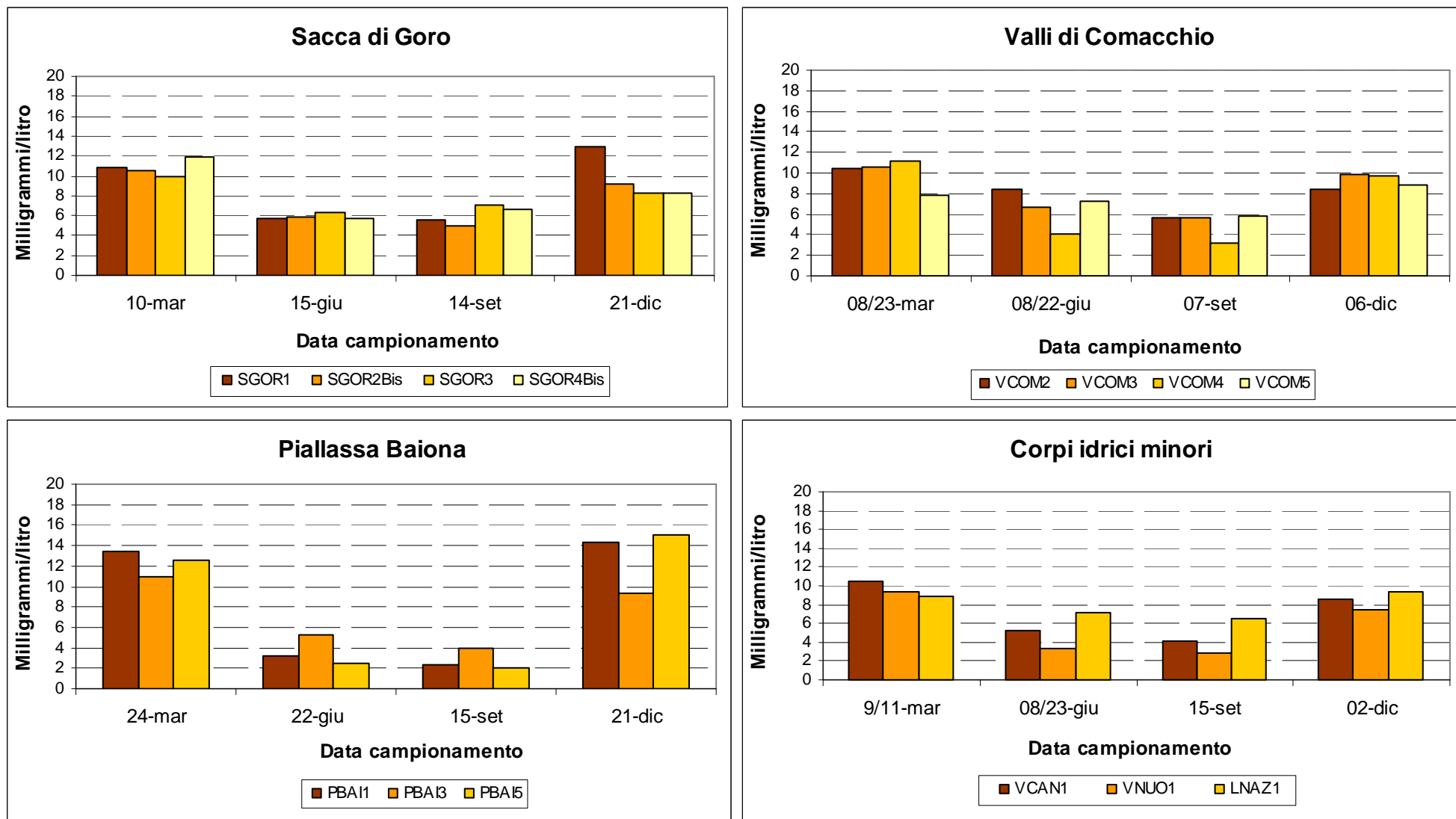
Figura 18 - Andamenti temporali dell'O.D. nei punti di campionamento dei corpi idrici di transizione: 2011
