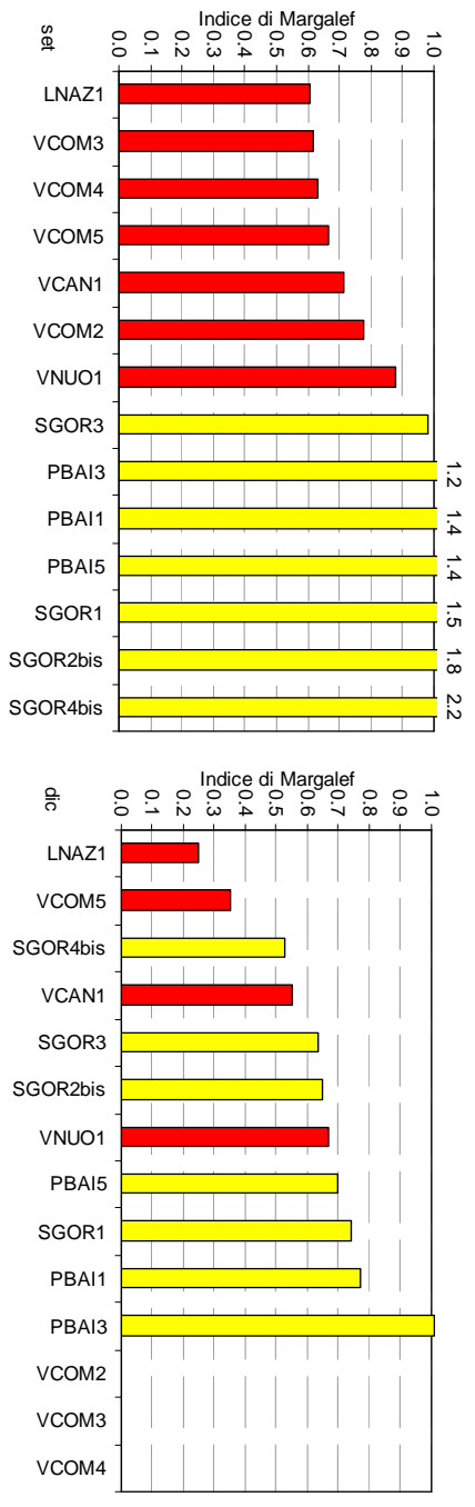
Figura 12 - Indice di Margalef per campagna di monitoraggio (lagune aperte , lagune chiuse ): 2012
