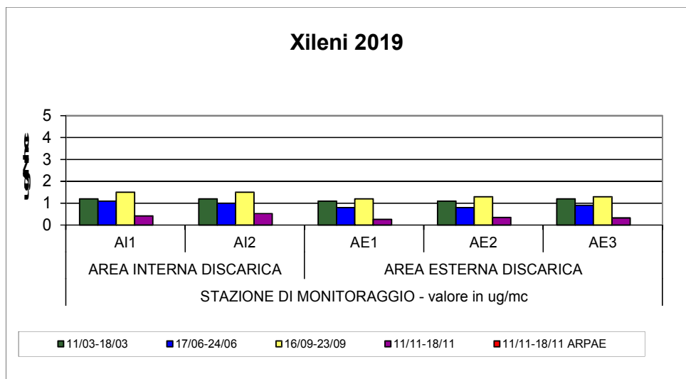
Grafico n. 5 – Andamento Xileni
