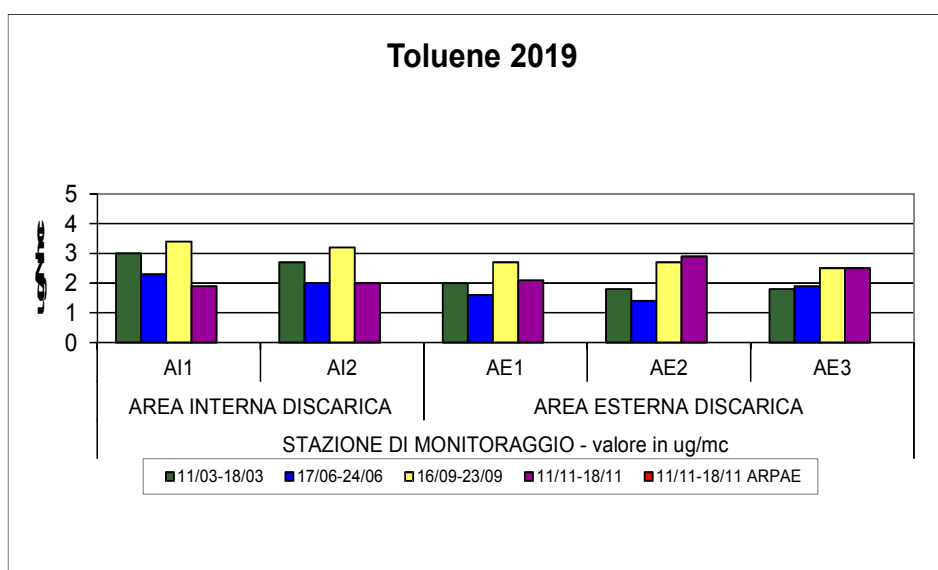
Grafico n. 4 – Andamento Toluene
