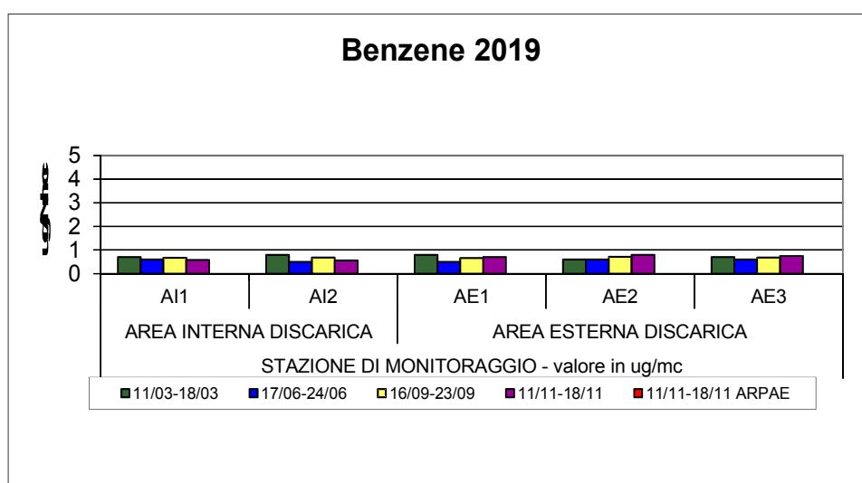
Grafico n. 3 – Andamento Benzene
