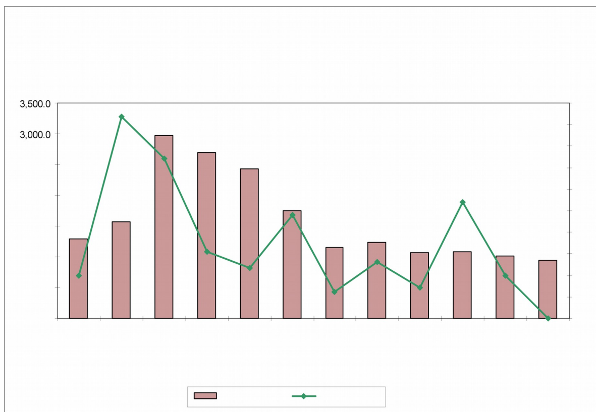
Grafico n. 1 – Andamento della produzione di percolato e piovosità in discarica Rio Riazzone nell'anno 2015
