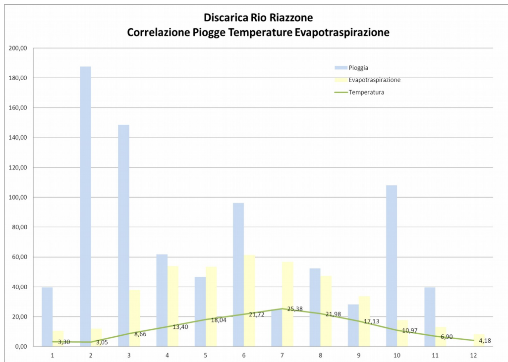
Grafico. n. 6 – Andamento di Temperature medie mensili, piovosità ed evapotraspirazione rilevati presso la Discarica di Rio Riazzone, anno 2015
