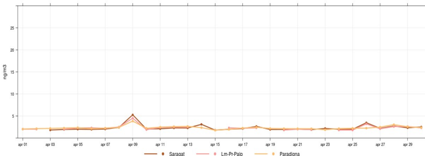
Figura 8: Hg, massimi giornalieri
