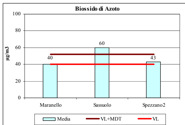
Figura 4.32: NO 2 -medie annuali
