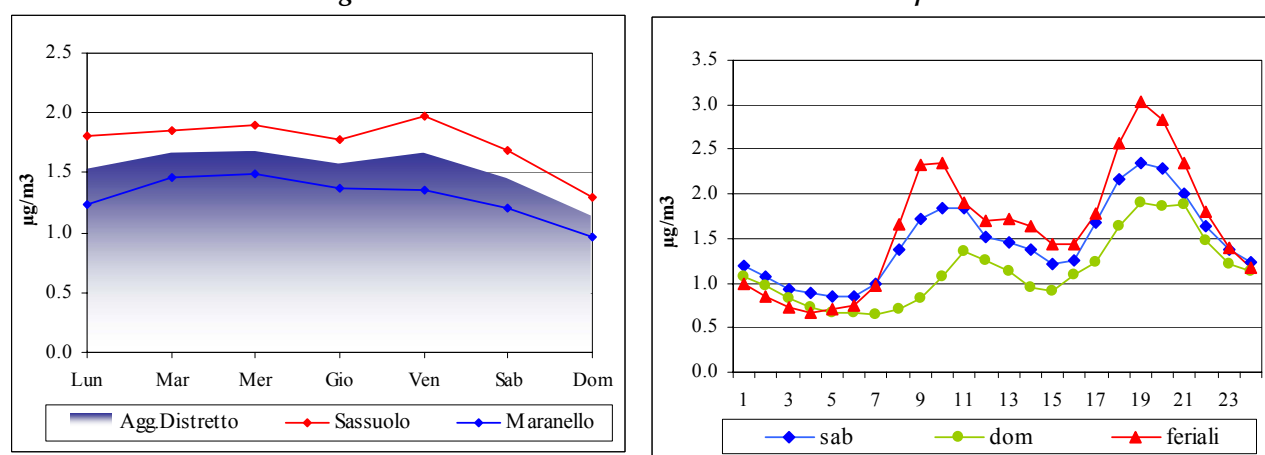
Figura 4.42: Benzene - giorno tipico annuale e giorno tipico feriale e festivo
