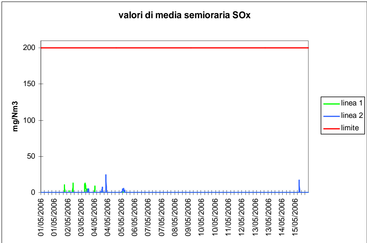
Figura 5: media semioraria SOx
