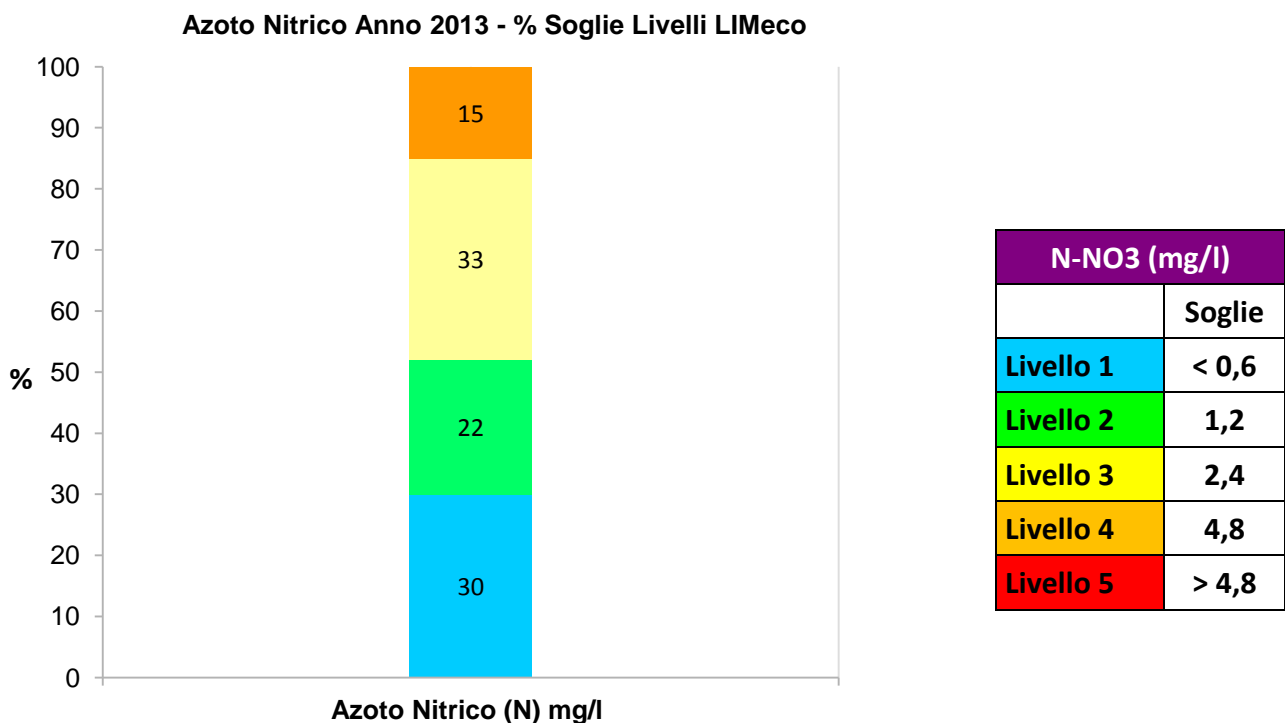
Grafico 19. AZOTO NITRICO- Percentuali Soglie Livelli LIM eco Anno 2013
