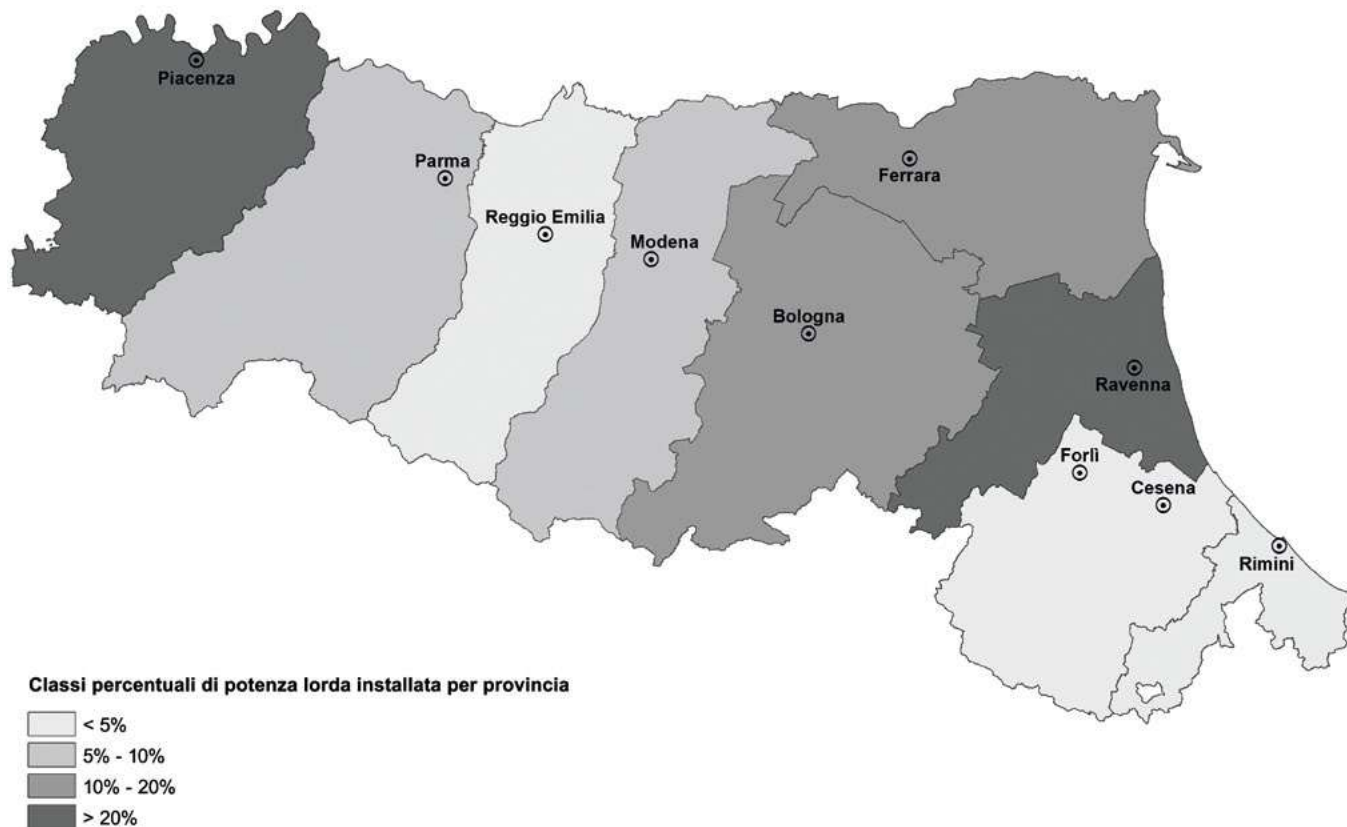
FIGURA 18 Classi percentuali di potenza lorda efficiente degli impianti di produzione di energia elettrica nelle province dell'Emilia-Romagna (anno 2017)
