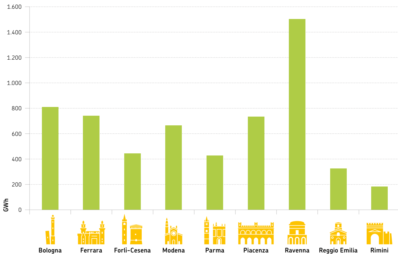
FIGURA 14 Produzione annuale lorda di energia elettrica da fonti energetiche rinnovabili in Emilia-Romagna, per provincia (anno 2017)
