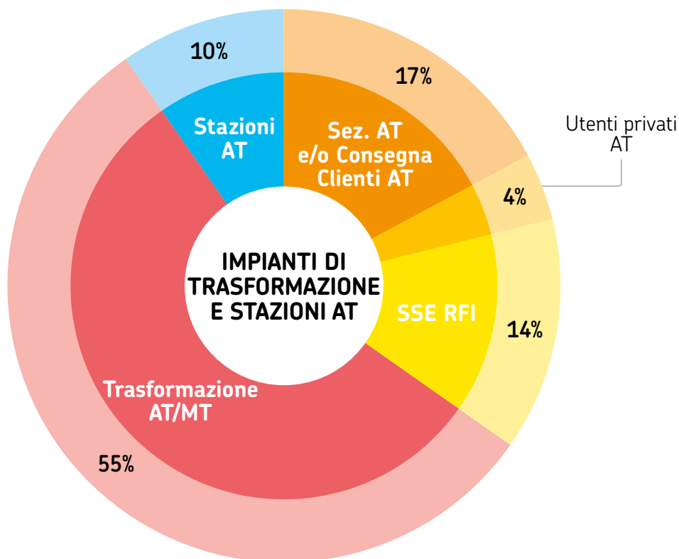
FIGURA 43 Impianti di trasformazione e stazioni AT presenti in Emilia-Romagna, distinti per tipologia (anno 2017)
